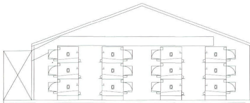
Dwarsdoorsnede
