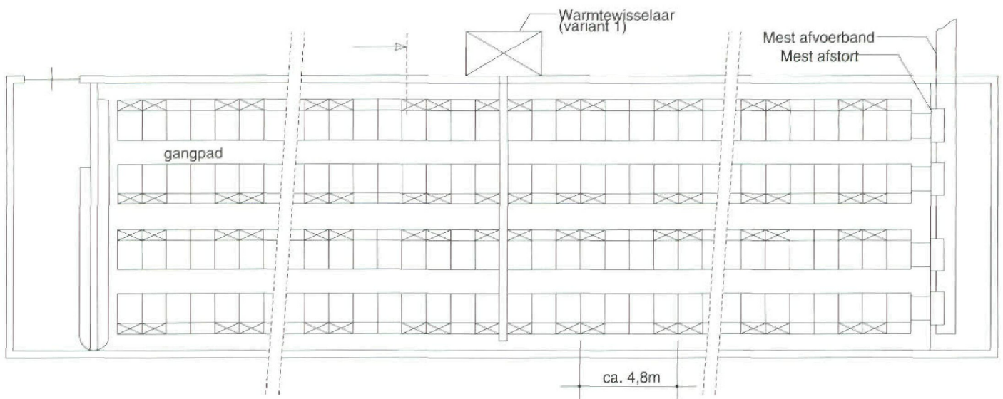
Plattegrond
