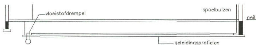
verdringings spoelsysteem doorsnede B-B
