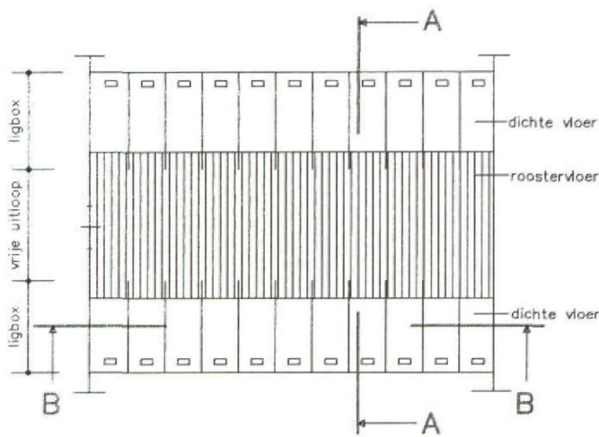
plattegrond dragende zeugen
