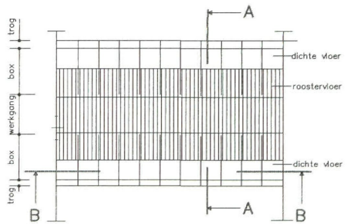
plattegrond guste zeugen
