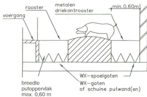
doorsnede B-B
