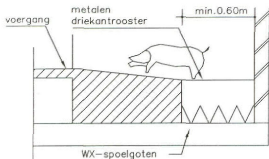
doorsnede A-A
