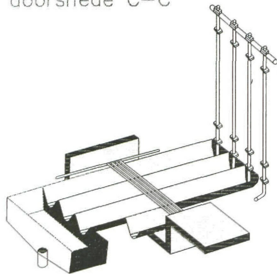
WX-spoelgotensysteem
